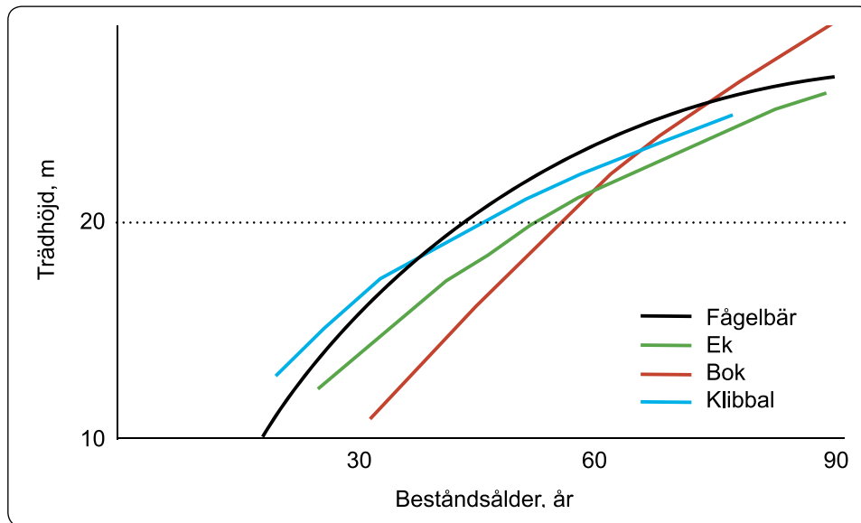
Figur ÄD9 Jämförelse av höjdtillväxten för fågelbär med andra lövträds- slag. 128
