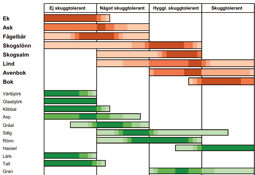
Figur ÄD4 De ädla lövträdens (rött) och andra trädslags (grönt) skuggtolerans. Schemat utarbetades med hjälp av flera av landets främsta lövskogsexperter. Den mörka delen av respektive trädslags område visar skuggtoleransen under större delen av omloppstiden. Ljusare delar markerar att trädslaget har en något annorlunda tolerans i till exempel plant- och ungdomsstadiet, och på ovanliga ståndorter. Källa: Rytter (1998). 46
