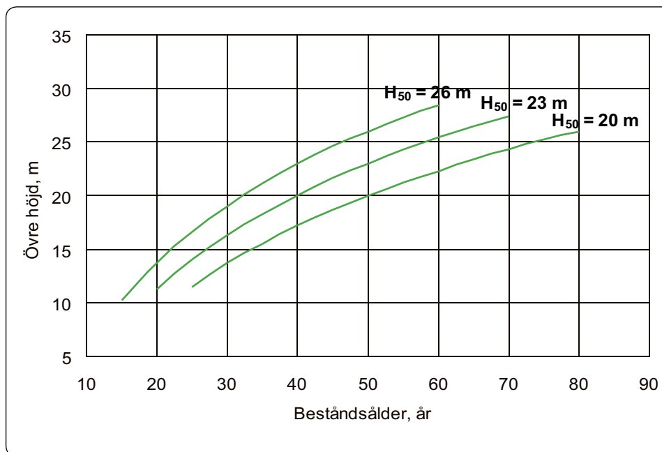
Figur ÄD10 Höjdtvecklingskurvor för fågelbär baserade på provytor i nordvästra Tyskland. Källa Röös (1993). 129
