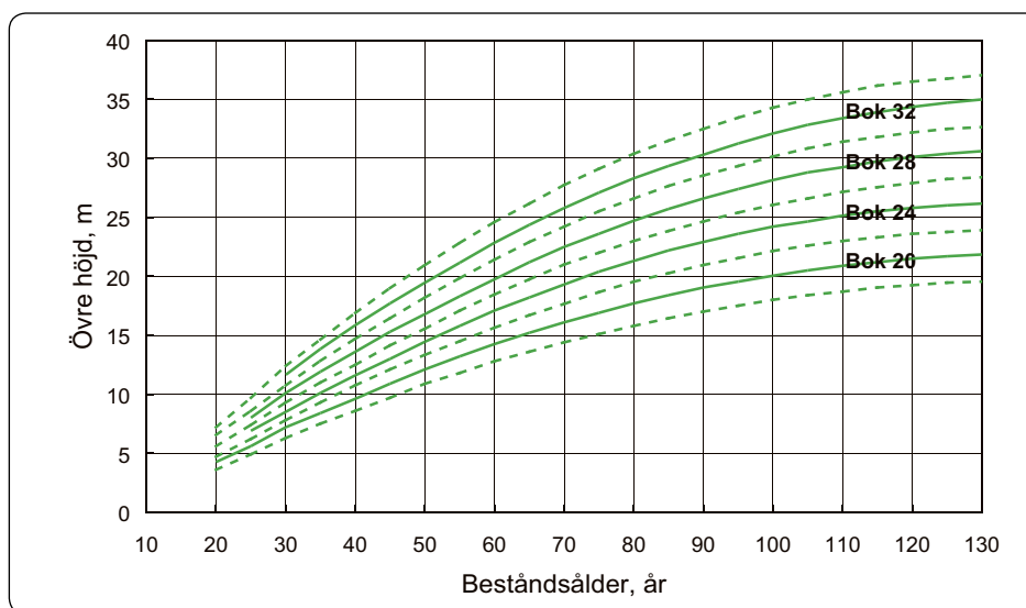
Figur ÄD7 Höjdutvecklingskurvor för bok baserade på 39 försöksytor i södra Sverige. 93
