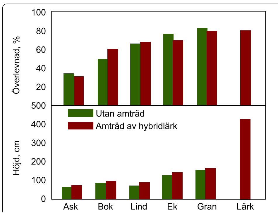
Figur ÄD17 Överlevnad och tillväxt av plantor av olika ädla lövträd samt gran fem år efter plantering innanför hägn med eller utan amträdkultur av hybridlärk. Överlevnaden skiljer sig kraftigt åt mellan olika trädslag och amkulturen har liten inverkan på överlevnad och tillväxt de första fem åren. Källa: Löf m.fl. 172
