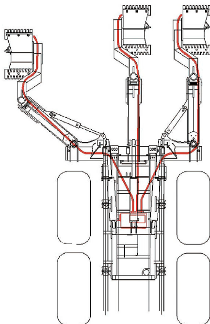
Figur S17 Princip för montering av såddapparater på ett 3-radigt variationsaggregat ( www.brackeforest.se ). En fläkt transporterar fröet i slangar till utsläppet längst ut på markberedningsaggregatet. Individuella frömatarhjul kontrollerar flödet av frön till varje såddkanal.
