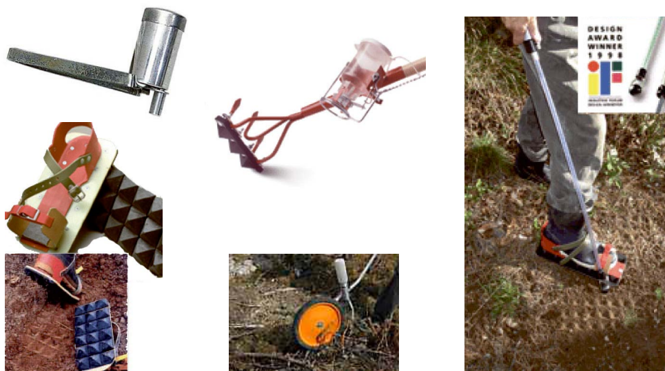
Figur S18 Såddkanna ( www.skogma.se ). Så-Dan klokratta utrustad med såddapparat och mikroprepareringsplatta. SilviCon såddrör för sådd på markberedda och mikropreparerade områden. Mikroprepareringssko för användning på markberedd mark ( www.silvitec.se ). Såddhjul för manuell radsådd med mikropreparering.
