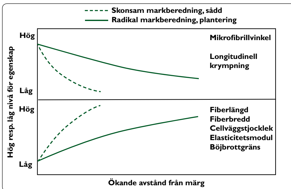
Figur S4 Vedegenskapers förändring med avstånd från märgen för tall planterad i glest förband efter radikal markberedning och för tall som såtts efter skonsam markberedning. 13
